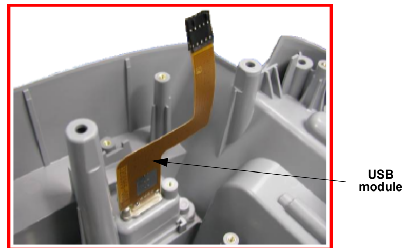
Figure 10.112—USB flex module
